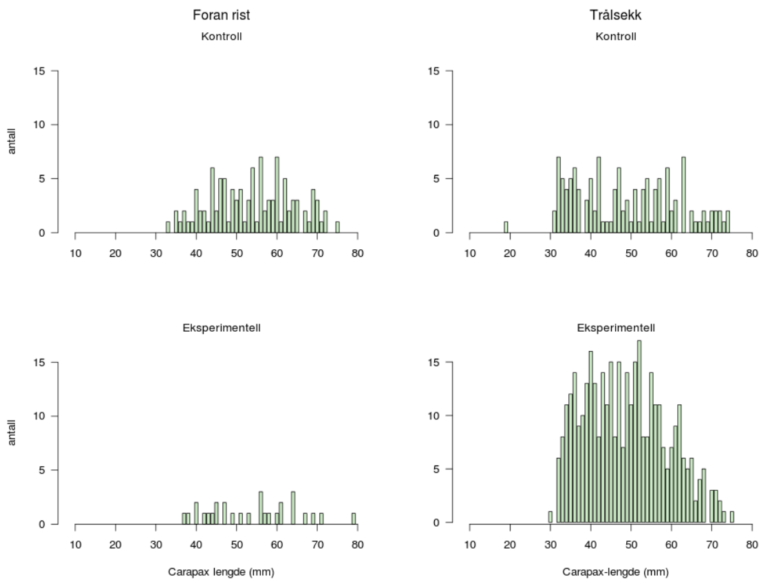
Figur 7. Lengdefordeling av kreps fanget fremfor rista og i trålposen for kontrollsiden (standard rista) og den eksperimentelle siden (rist med krepsehull).
